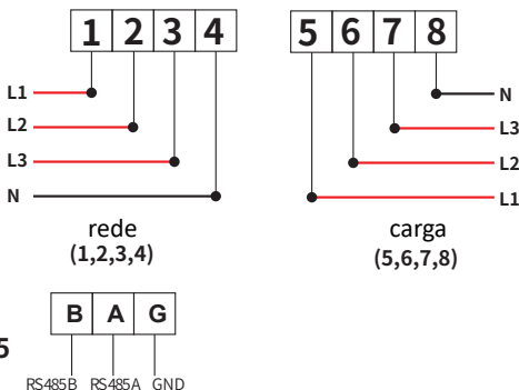
Figura 7.18 Medidor Eastron
