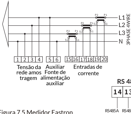
Figura 7.5 Medidor Eastron
