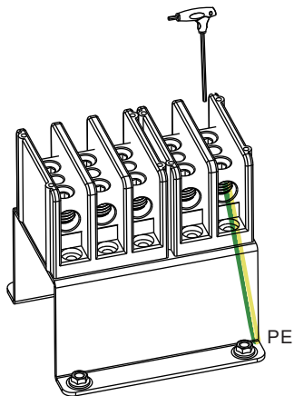
Figura 5.8 A instalação do condutor terra na carcaca
