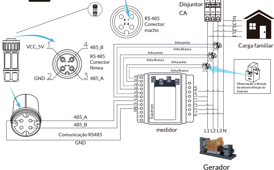
Figura 7.8 Diagrama de conexão do medidor Eastron
